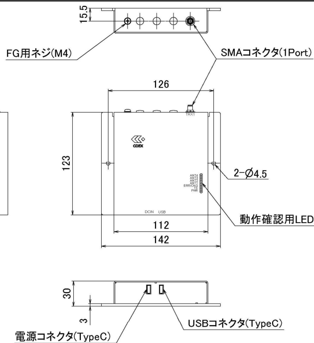
各部の名称および外形寸法
